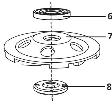
Hiomalaikan asentaminen
