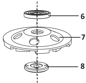
Montage/Demontage der Diamant-Schleifscheibe
